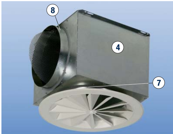
Anschlussart D, \dot{V} -Drossel im Anschluss-Stutzen
