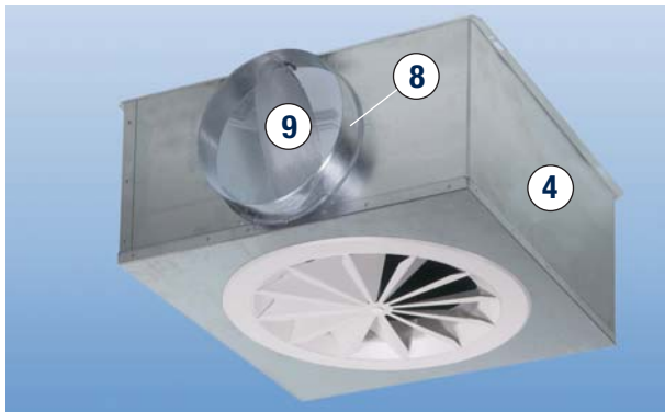
Anschlussart E, \dot{V} -Drossel im Anschluss-Stutzen
