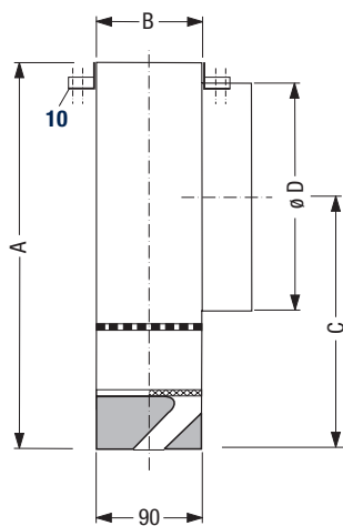
Schnitt A – A Anschlusskasten, dargestellt ohne akustische Auskleidung, ohne \checkmark -Drossel
