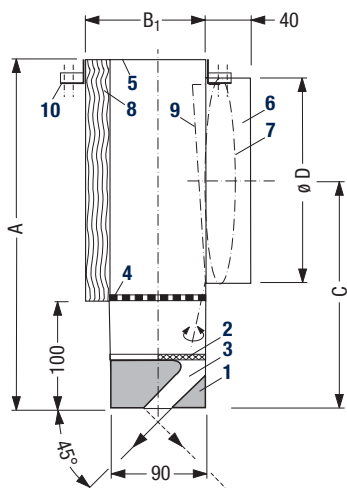
Schnitt A – A Anschlusskasten, dargestellt mit akustischer Auskleidung, und \checkmark -Drossel 7 im Anschluss-Stutzen, vom Raum her verstellbar
