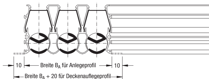
Bild 8: Darstellung der Eckwinkel für IN-V2; 1- bis 4-reihig (dargestellt ist die 3-reihige Ausführung)
