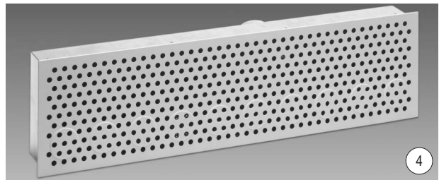
Fächerauslässe für Zuluft und Abluft mit gelochter Frontplatte, Strahlbündelelemente in zweireihiger Anordnung ③ sowie Kombiniertes Fächerauslass für Zuluft und Abluft ④ mit gelochter Frontplatte und Strahlbündelelemente im unteren Zuluftteil. Die Strahlbündelelemente können zur Veränderung der Ausblasrichtung manuell gedreht werden.
