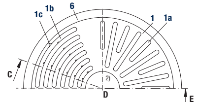
DN 200 - Draufsicht bei Einbau mit Spanneinsatz
