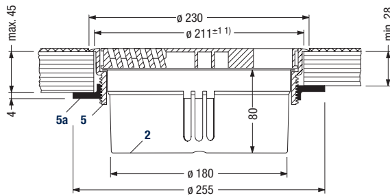
DN 200 mit Spanneinsatz und Spannmutter, Verteilkorb VK
