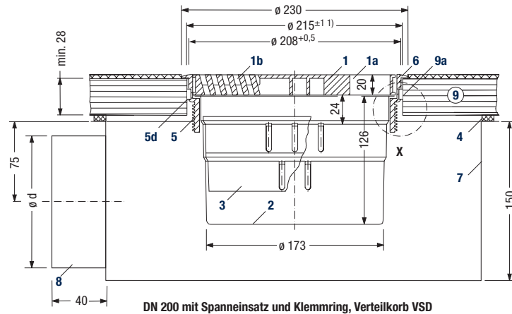
DN 200 mit Spanneinsatz und Klemmring, Verteilkorb VSD
