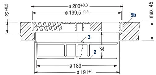
DN 200 Einbau in Stufenbohrung, Verteilkorb VND
