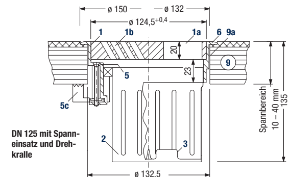
DN 125 mit Spanneinsatz und Drehkrallen
