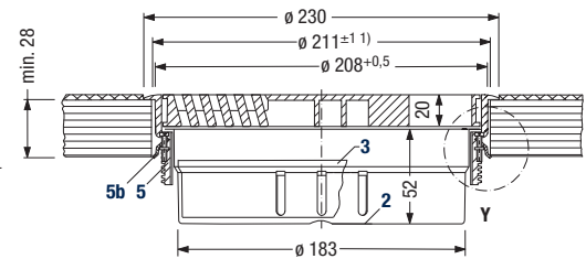
DN 200 mit Spanneinsatz und Spreizkrallen, Verteilkorb VND
