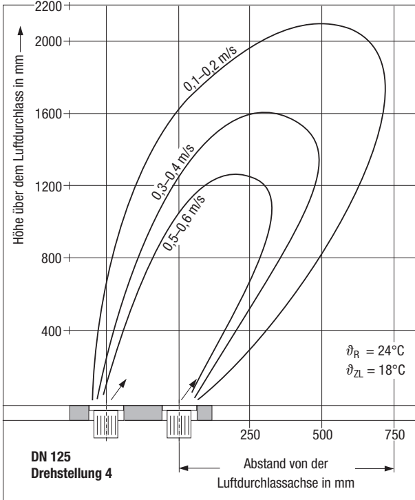
Bild 5: Verlauf der Strahlgeschwindigkeit für DN 125, Drehstellung 1 und 4, Volumenstrom 50 m³/h je Luftdurchlass
