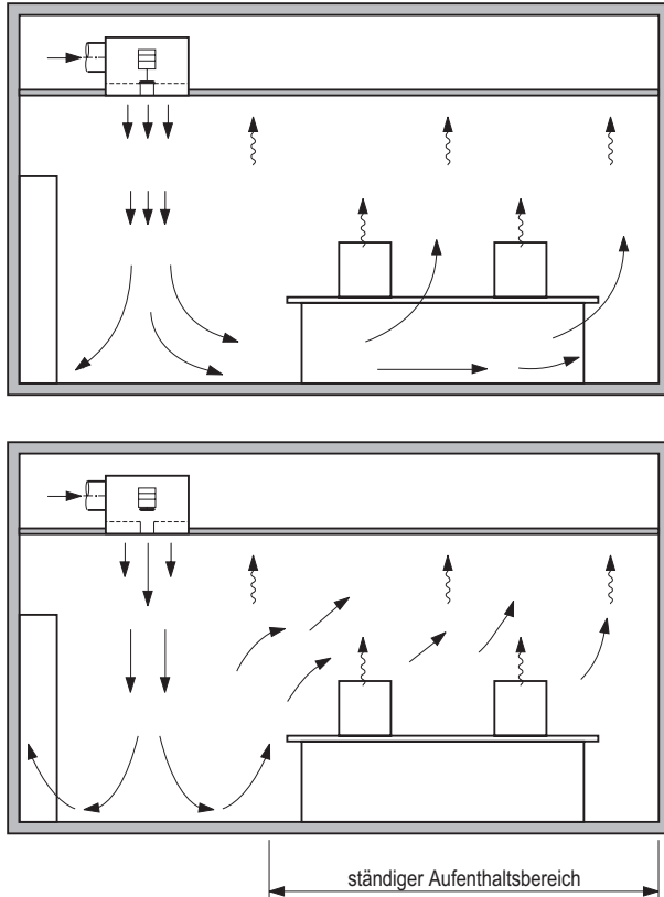
Bild 3: Charakteristik der Raumluftströmung, dargestellt mit dem Verstellbaren Deckenquellauslaß, oben: Kühlfall, unten: Heizfall.
