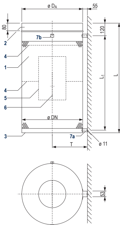
Bild 1: Baugrößen und Abmessungen
