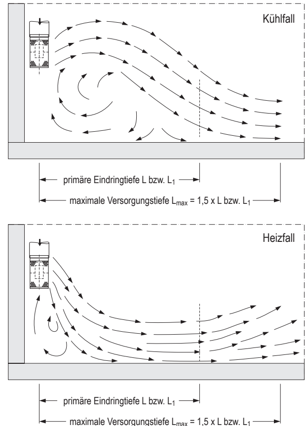
Bild 6: Primäre Eindringtiefe und maximale Versorgungstiefe der Zuluftstrahlen bei Anordnung über dem Aufenthaltsbereich
