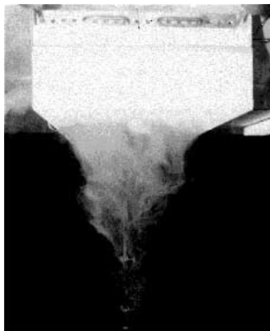
Bild 5: Typisches Strömungsbild unterhalb eines passiven Deckenkühlkonvektors
