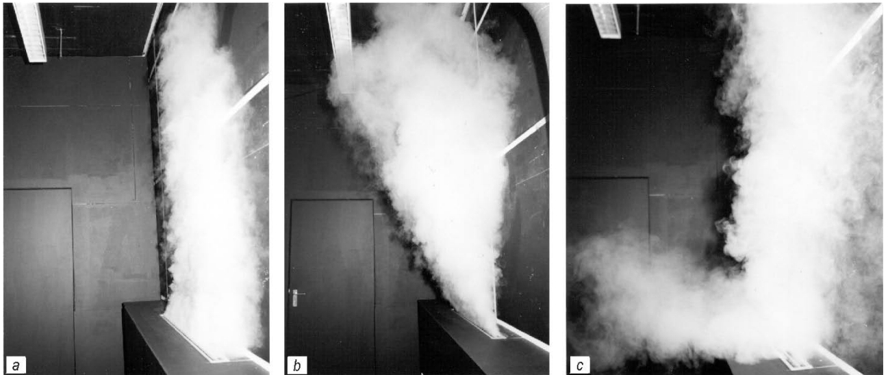
Bild 4: Zuluffführung über verstellbaren Induktivauslass, durch Rauchprobe sichtbar:
