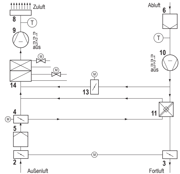
Bild 2: Schema luftechnische Funktion
