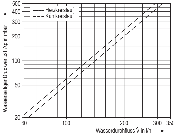
Bild 3: Druckverlust des Wärmeaustauschers im Lüftungsgerät
