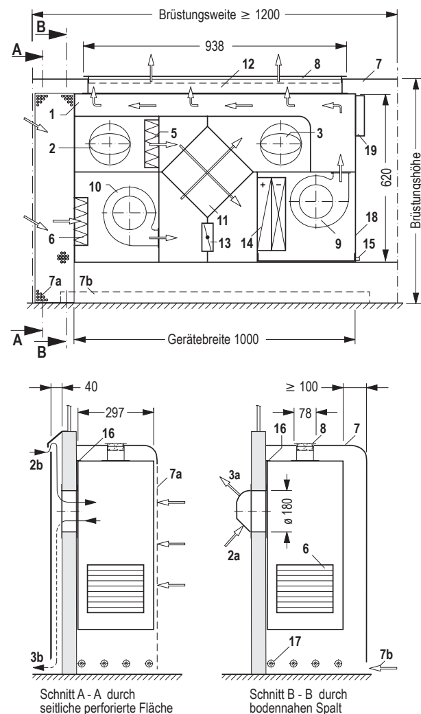
Bild 1: Hauptabmessungen sowie Darstellung der Abluftöffnungen in der bauseitigen Brüstungsverkleidung; das Bild zeigt ferner als Beispiel die verdeckten Ansaug-/Ausblasöffnungen (2b und 3b) und die sichtbare Ausführung (2a und 3a); Wasseranschluss rechts 18, Regeleinheit und Elektroanschluss 19
