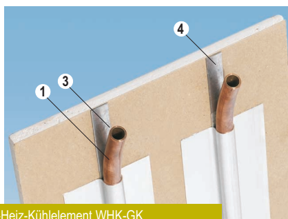
Wand-Heiz-Kühlelement WHK-GK Anschlussseite
