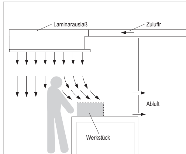
Strahlcharakteristik Laminarauslaß
